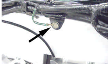
アース線をエアクリーナーステー部のボルトでフレームに取り付ける。
