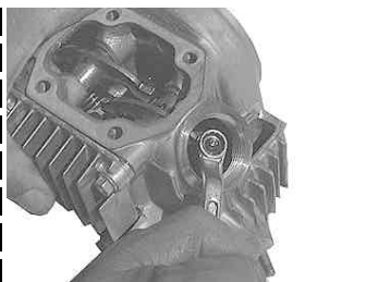
シリンダーヘッドに組まれているロッカーアームのタペットナットとボルトを取り外す。タペットナットを緩めた時点でタペットボルトをナットと一緒に取り外す。
