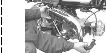
アース線をエアクリーナーステー部のボルトでフレームに取り付ける。
