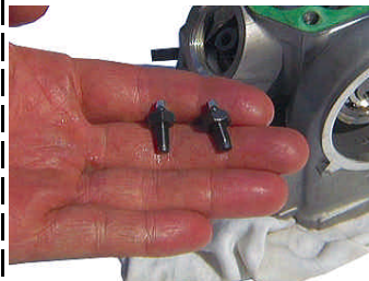
カムチェーンを引っ張りながらガイドローラーを付ける。
