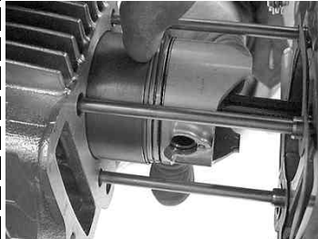
シリンダーをピストンリングの合い口がずれない様しながら指で押し少しづつはめる。ここは難易度が高いです。がんばってください。
