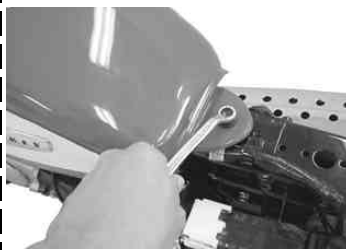
フューエルタンクをフレームにとめているボルトを取り外す。
