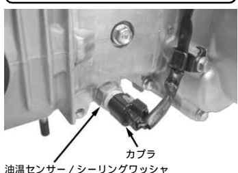
カブラ 油温センサー / シーリングワッシャ
