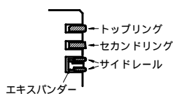
ピストンリング断面形状
