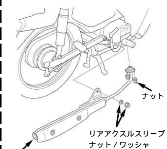
エキゾーストマフラー
