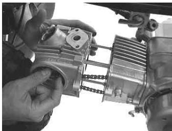
ヘッドガスケットを取り付ける。
