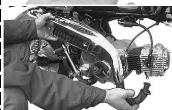
ワイヤーハーネスをフレームの下側になるように移動させる。
