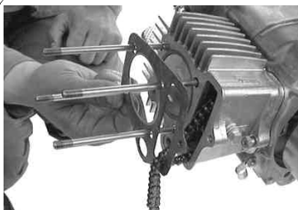
ヘッドガスケットを取り付ける。
