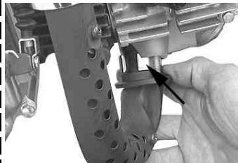
フランジのカラー2個を取り外し外側に引く様にしてマフラーを車体から取り外す。
