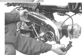
使用工具 ボックスレンチ 10 mm エクステンションバー 小 規定トルク 12 N・m (1.2 kgf・m)
