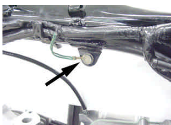
アース線をエアクリーナーステー部のボルトでフレームに取り付ける。
