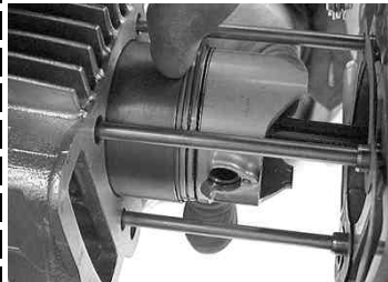
シリンダーをピストンリングの合い口がずれない様になりながら指で押し少しづつはめる。ここは難易度が高いです。がんばってください。
