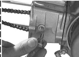
ガイドローラーボルトを取り付ける。(指で閉まる程度まで仮止め)
