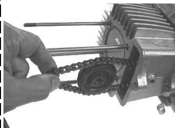
カムチェーンを引っ張りながらガイドローラーを付ける。
