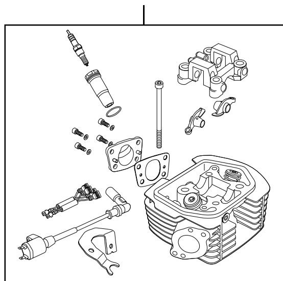
01-03-0772 ツインスパークスーパーヘッドST-3キット
