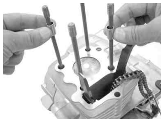
シリンダーヘッドのマニホールド取り付け面のガスケットカスをスクレーパーやカッターナイフ等できれいに取り除きます。
