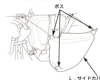
L. サイドカバー
