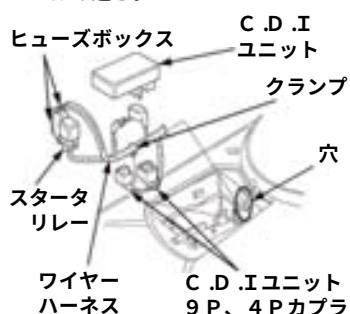
9P、4Pカブラ
