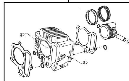
01-04-0107 シリンダーキット111ccシリンダー
