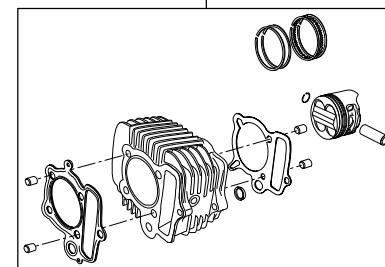
01-04-8008 シリンダーキット88cc Vシリンダー
