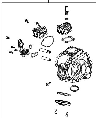
01-03-0116 スーパーヘッド4バルブ+Rキット
