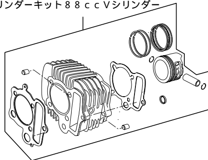
01-04-8088V シリンダーキット88cc Vシリンダー
