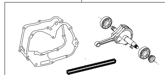
01-10-8432 ストロークアップクランクキット (50ストローク)
