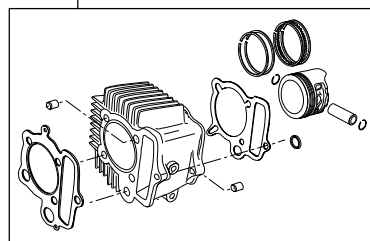
01-04-7106H シリンダーキット106cc Hシリンダー
