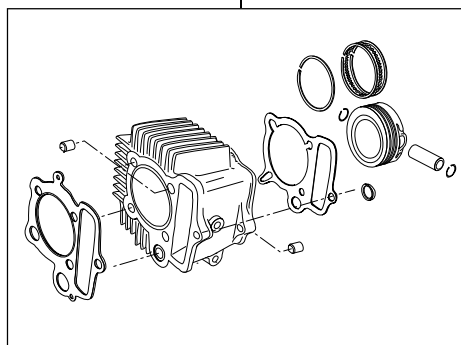
01-04-0127 シリンダーキット125cc SCUTシリンダー
