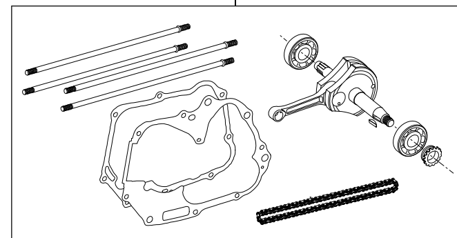
01-10-0118 ストロークアップクランクキット(48.9ストローク)
