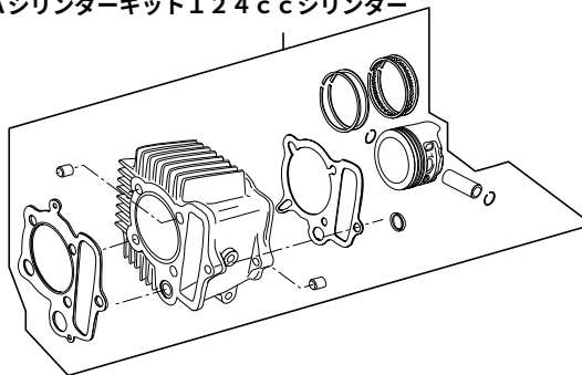
01-04-8224H HAシリンダーキット124ccシリンダー
