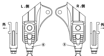
チェーンスライダーCOMP.組み付け図
