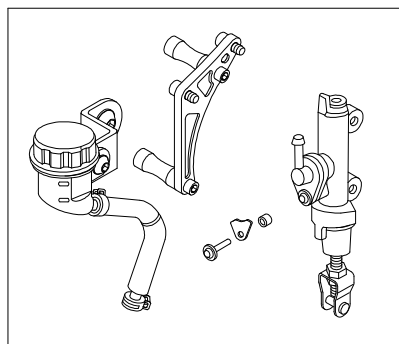
リアマスターシリンダー
